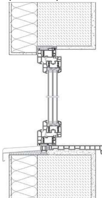
Ryc. 2. Prawidłowy montaż okna.
